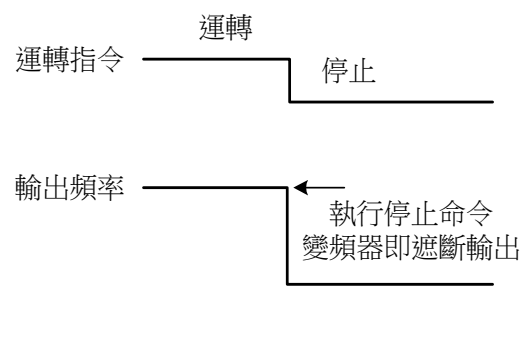
圖 4-5-2：自由運轉停止(2-03=1)
