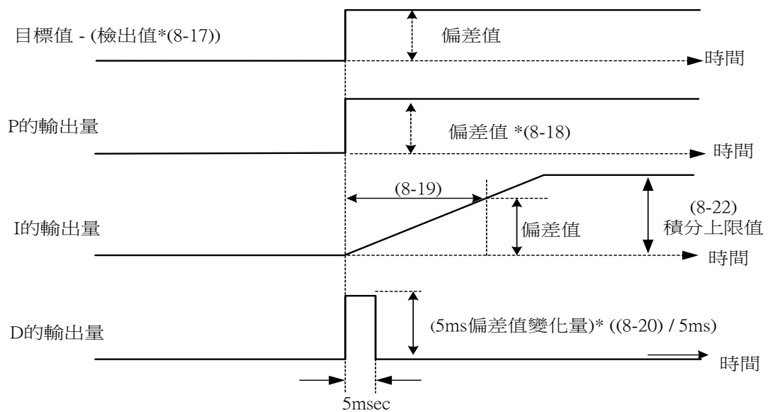
圖 4-24：PID 控制架構圖 (當(8-16)=1, PID 控制有效時)
