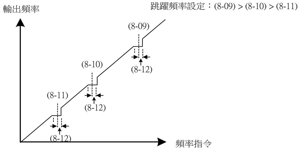
圖 4-22：跳躍頻率控制
