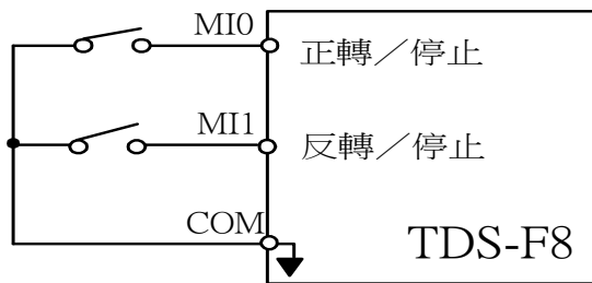
圖 4-10： 2 線式操作接線
