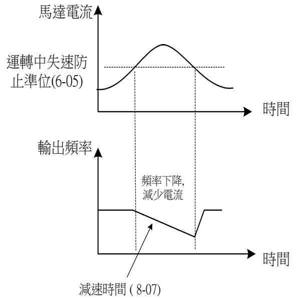
圖 4-16-2：運轉中失速防止機能
