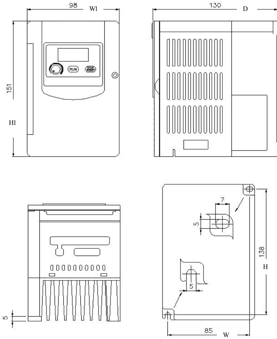
圖 1-6: 外形尺寸圖
