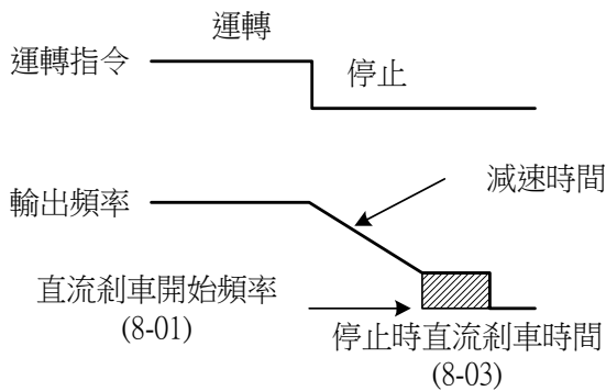
圖 4-5-1：減速停止(2-03=0)
