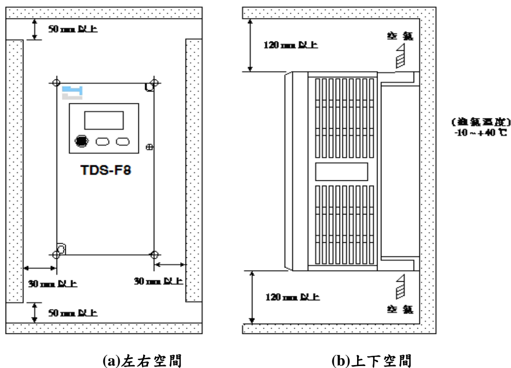
圖 1-2 TDS-F8 安裝空間圖
